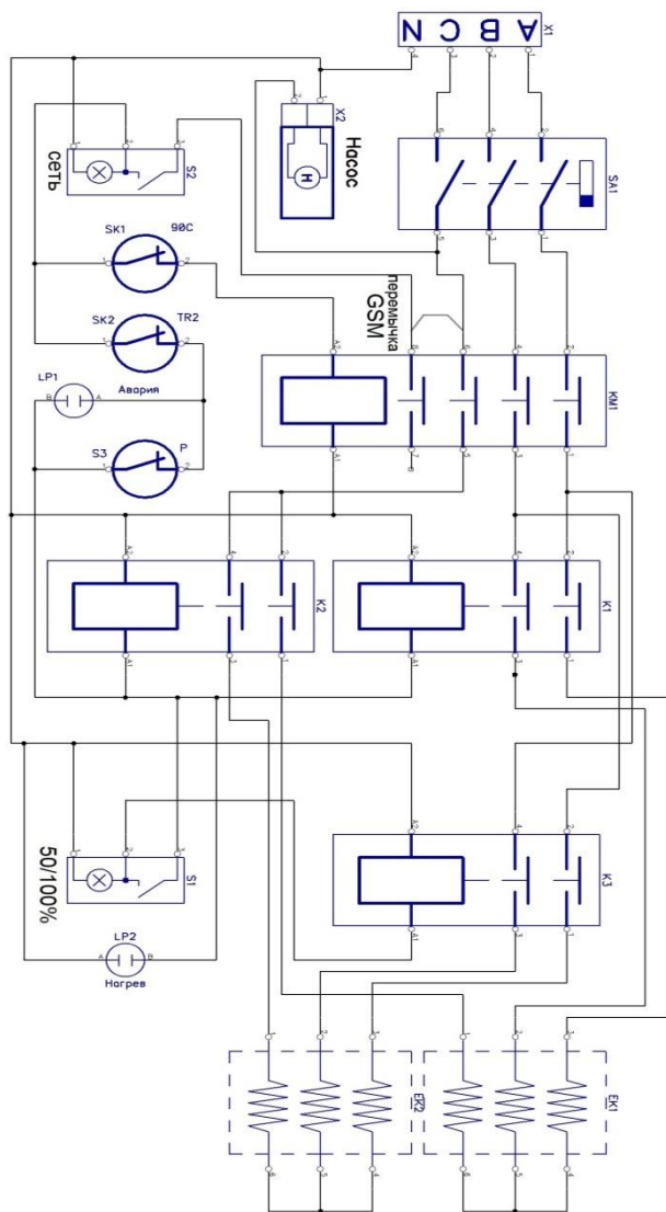
СХЕМА ЭЛЕКТРИЧЕСКАЯ ПРИНЦИПИАЛЬНАЯ ЭЛЕКТРОКОТЛА ТHERMICS 002-2VR
